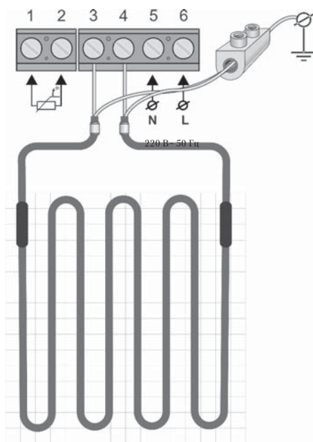
Рис. 3. Схема подключения одножильного нагревательного мата
