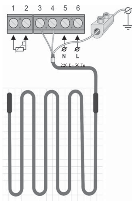
Рис. 4. Схема подключения двухжильного нагревательного мата
